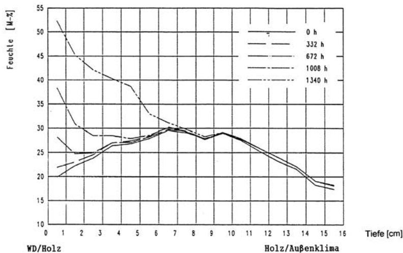
Bild 8 Feuchteverlauf im Holz/Eiche über den Querschnitt während der Winterperiode
