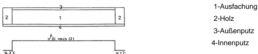
Bild 1 Schnitt Außenwandbauteil/Oberflächentemperaturverlauf "naiv"
