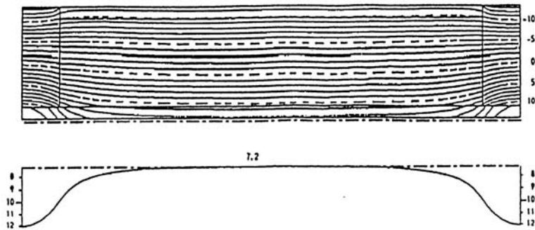
Bild 2 Temperaturfeld Außenwandbauteil/Oberflächentemperaturverlauf
