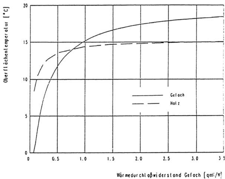
Bild 3 Oberflächentemperatur im Bereich Gefach und Holzbauteil
