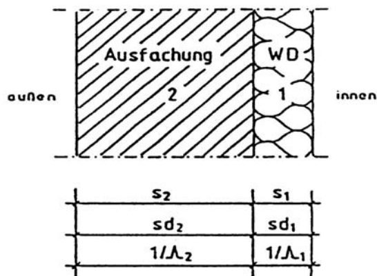
Bild 12 Schnitt Fachwerkaußenbauteil im Bereich Gefach
