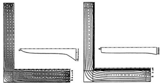
Bild 5 Fachwerkaußenkante Temperaturfeld/Oberflächentemperatur
