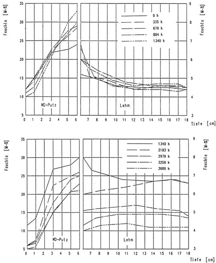
Bild 10 Feuchteverlauf im Gefach über den Querschnitt während Winter- und Sommerperiode
