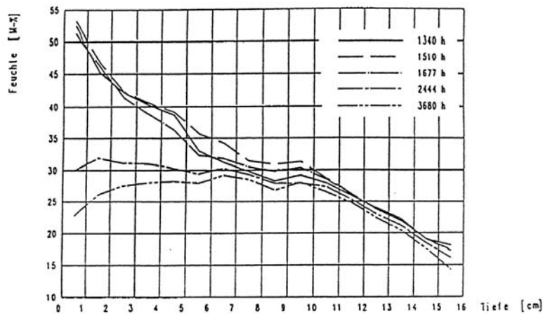
Bild 9 Feuchteverlauf im Holz/Eiche über den Querschnitt während der Sommerperiode
