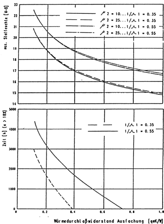
Bild 13 Maximale Stofffeuchte Holz und deren zeitliche Überschreitungsdauer von 18 M-%
