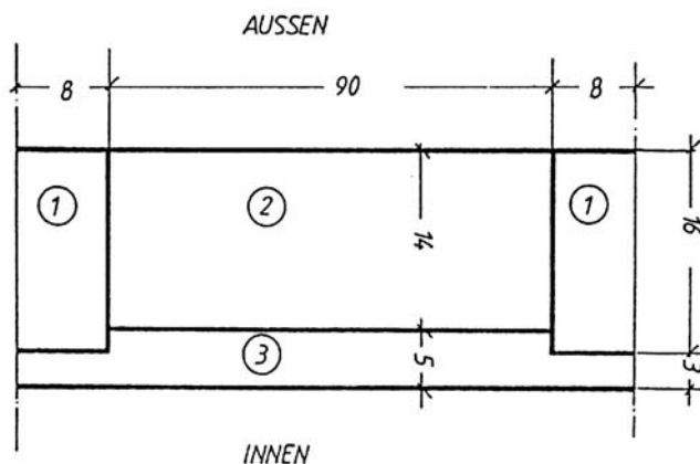
Bild 11 Fachwerkaußenbauteil
