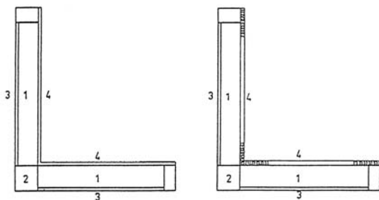
Bild 4 Schnitt Außenkante Gefach homogen und Wärmedämmschicht innen
