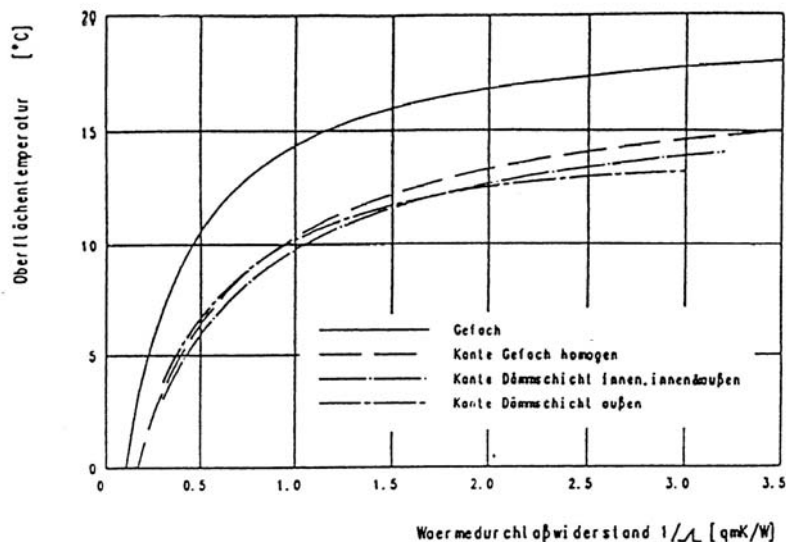
Bild 6 Oberflächentemperatur im Bereich Kante und ungestörtes Gefach in Abhängigkeit der Art und Lage der Wärmedämmschicht
