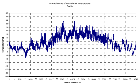
室外气温的年变化曲线图
