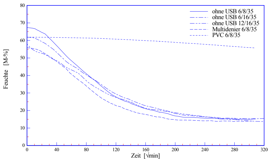
Bild 1 Rücktrocknungsverhalten Holz
