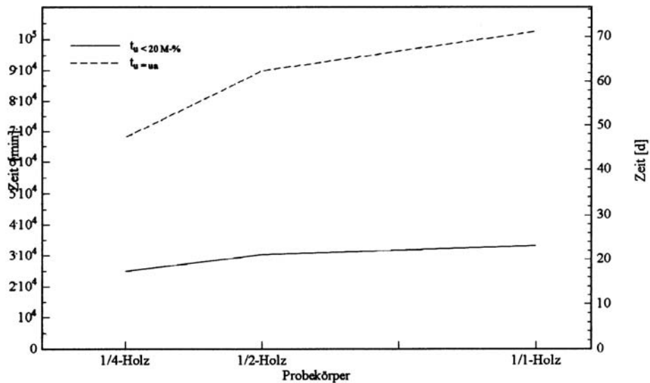
Bild 2 Trocknungsgeschwindigkeit in Abhängigkeit der Querschnittgröße
